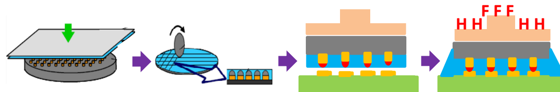
(d) TCB with High-Force of C2 Bumps (NCF)
